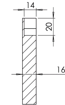
SECCIÓN A-A
